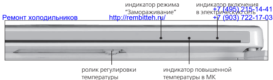
Рисунок 6 — Световая индикация холодильника однокомпрессорного (со звуковой сигнализацией)
